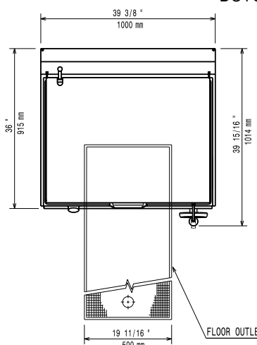
Boven aanzicht
